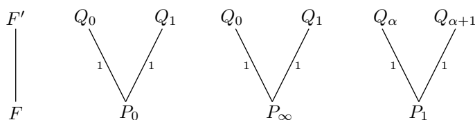
Gráfica 2.1: Descomposición de algunos ceros y polos de K(x)
