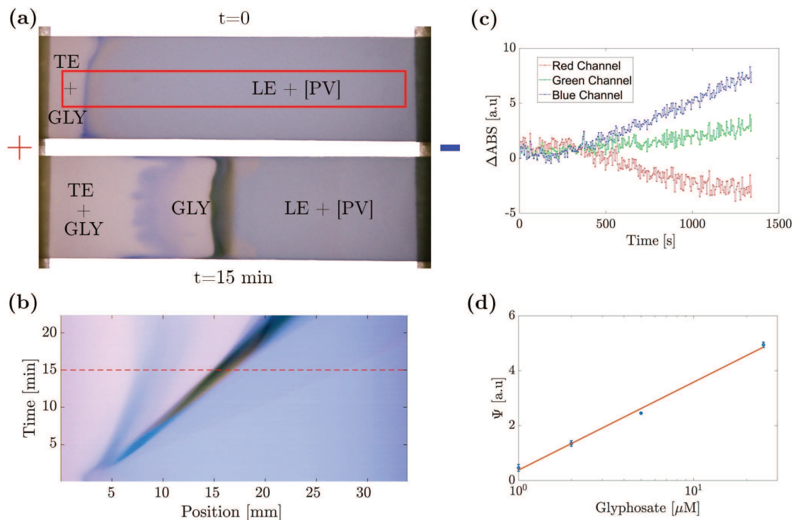
Figura 3.8: Resultados de detección de GlyP en el e- \mu PAD mediante ITP con detección colorimétrica. (a) Fotografías al inicio y a los 15 minutos, con el área de análisis en rojo. (b) Matriz espacio-temporal mostrando la dinámica del sistema. La línea punteada indica la imagen promedio vertical (a), en t=15 min. (c) Valores de \Delta ABS integrados espacialmente, por canal, a lo largo del tiempo. (d) Curva de calibración para múltiples concentraciones de GlyP (1, 2, 5 y 25 \mu M) usando el índice de absorción integrada \Psi .
