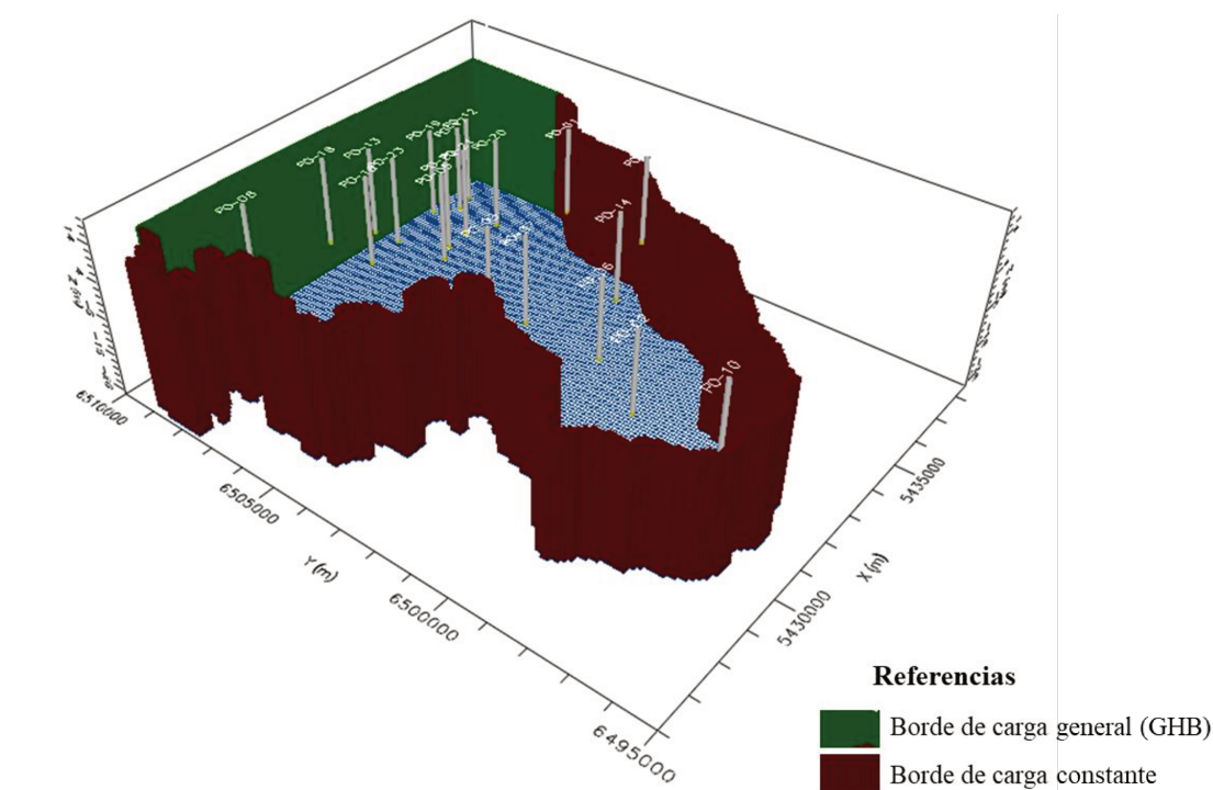
Figura 6.7.- Condiciones de borde asignadas
