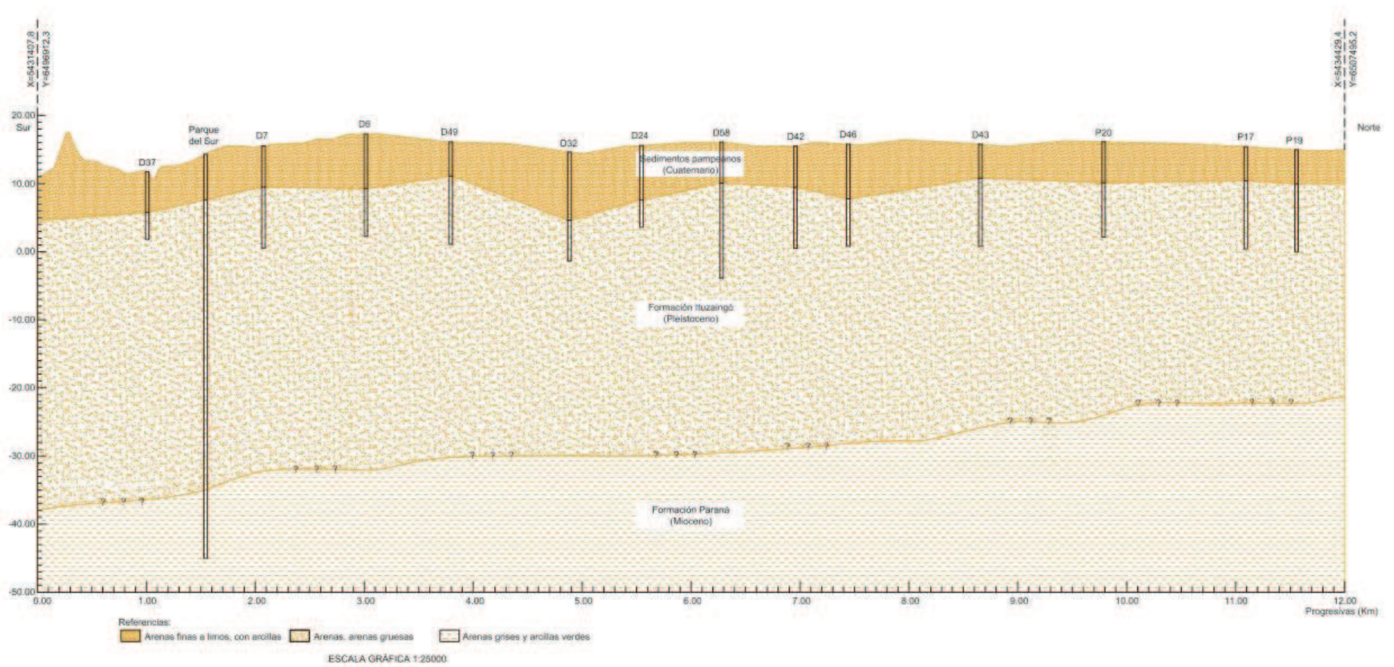
Figura 2.12.- Transecta D-D'. Dirección sur-norte
