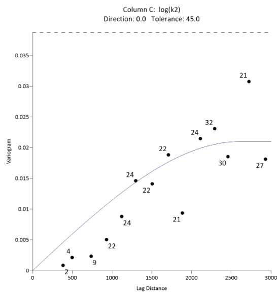
Figura 5.18a.- Dirección O-E
