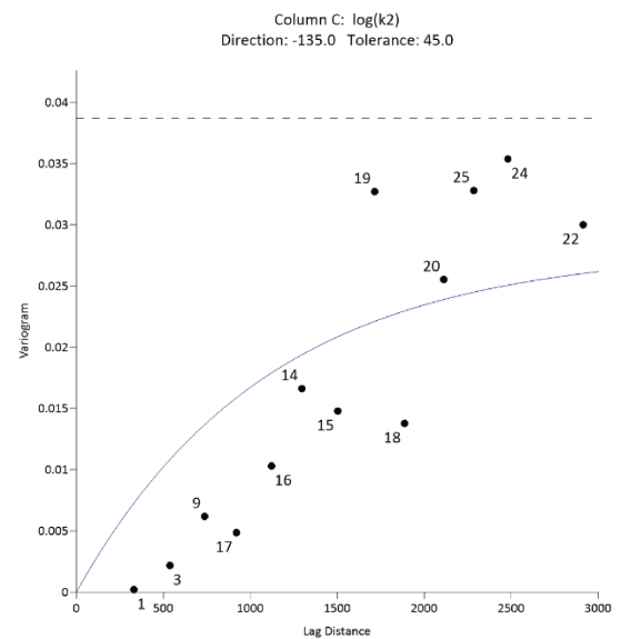
Figura 5.17d.- Dirección SO-NE
