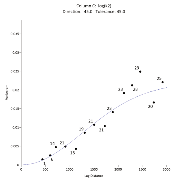
Figura 5.19b.- Dirección NO-SE
