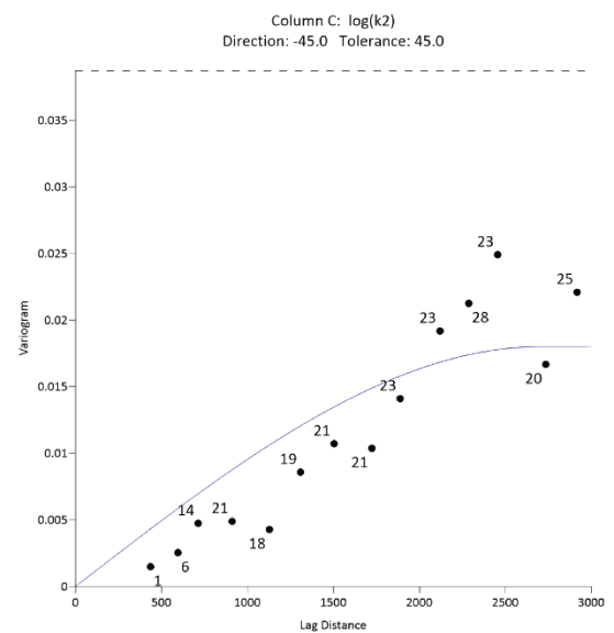
Figura 5.18b.- Dirección NO-SE
