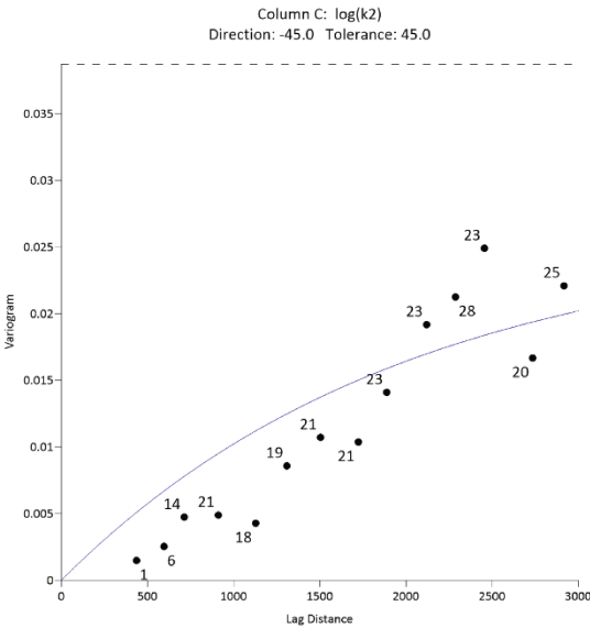
Figura 5.17b.- Dirección NO-SE
