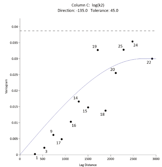
Figura 5.18d.- Dirección SO-NE
