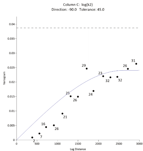
Figura 5.18c.- Dirección N-S
