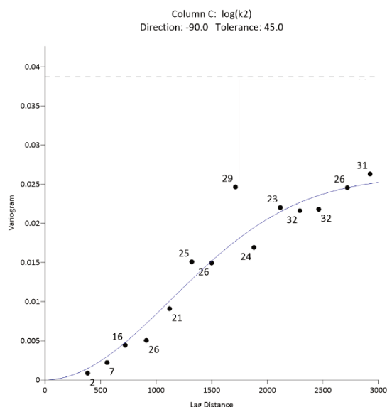
Figura 5.19c.- Dirección N-S
