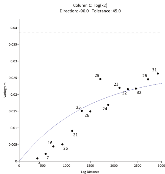
Figura 5.17c.- Dirección N-S
