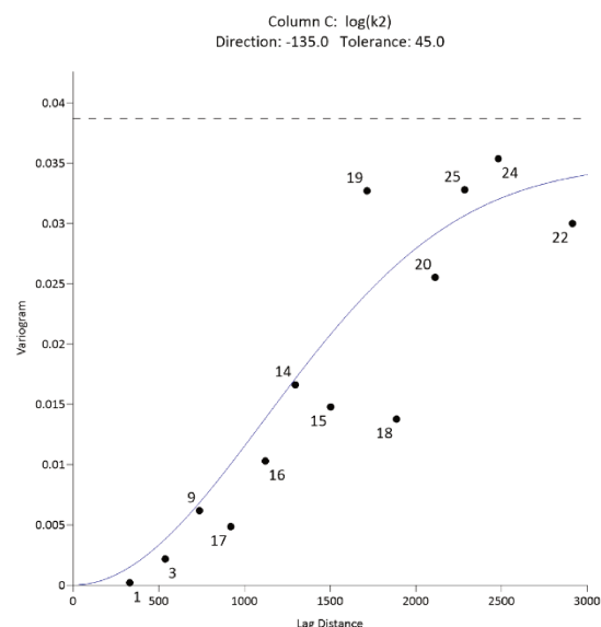
Figura 5.19d.- Dirección SO-NE
