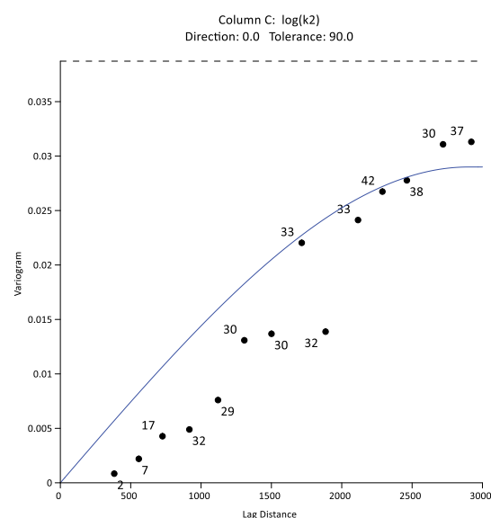
Figura 5.13b.- Opción 2: Esférico
