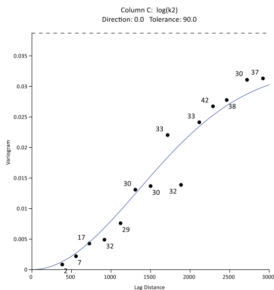
Figura 5.13c.- Opción 3: Gaussiano
