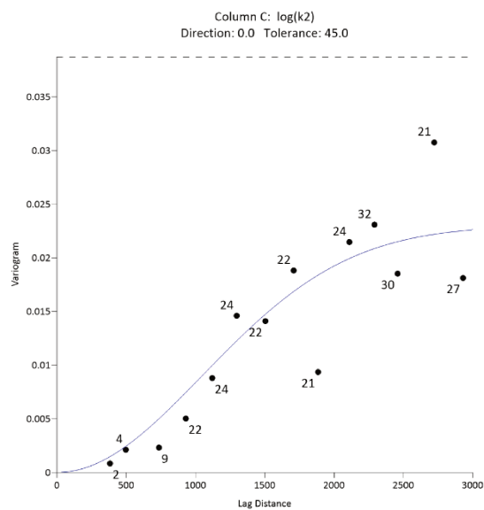
Figura 5.19a.- Dirección O-E
