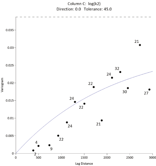
Figura 5.17a.- Dirección O-E
