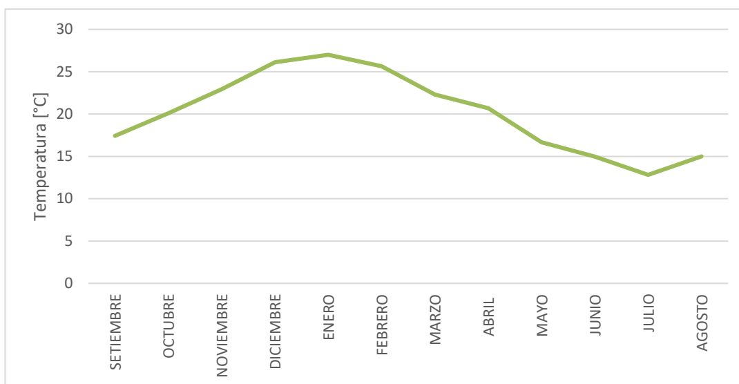
Figura 2.3.- Distribución de temperaturas medias mensuales. Período 2013-2023.
