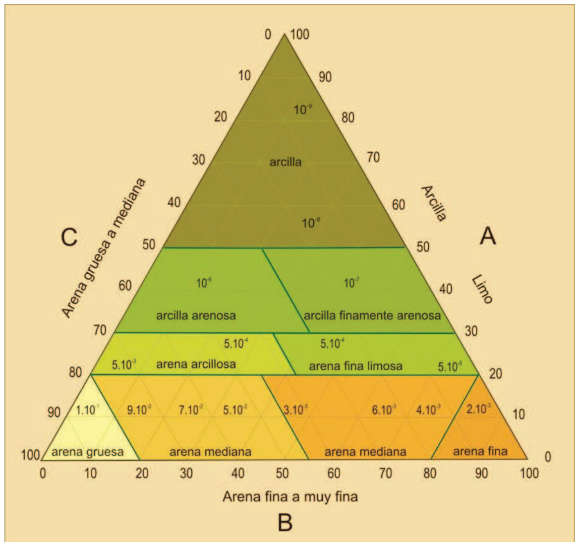
Figura 3.5.- Gráfico para la determinación de K [ \text{cm/s} ] según composición granulométrica. Modificado de Fili y Kolomi (inérito)
