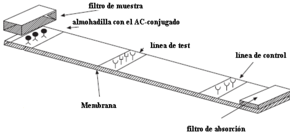
Figura 4. Componentes de un dispositivo de inmunocromatografía de flujo lateral en un paso (fuente: Van Herwijnen, 2006).
