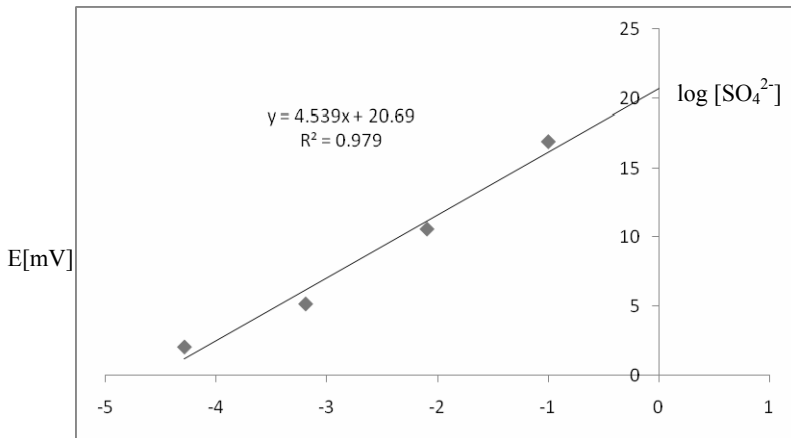
Figura 4. Curva de calibración típica de la respuesta del potencial medido con el logaritmo de la concentración de sulfatos en el medio.
