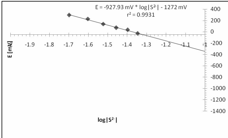
Figura 3. Muestra una curva de calibración típica de la respuesta del potencial medido con el logaritmo de la concentración de sulfuros en el medio.
