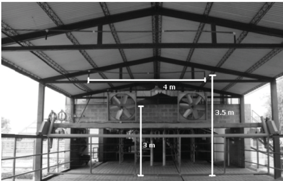
Fig. 2: Corral de espera con aspersores y ventiladores del INTA EEA Rafaela
