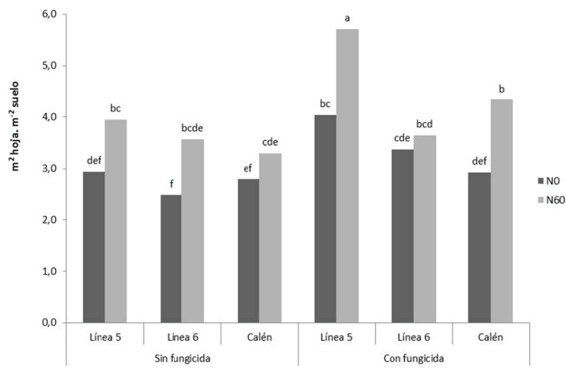
Figura 3: Media de los valores de IAF ( m^2 hoja. m^2 suelo) en EC3.9 para la interacción Fungicida x Fertilizante x Genotipos, en un ensayo con dos tratamientos de fungicidas, dos dosis de fertilización nitrogenada y tres genotipos de avena. Sin fertilizante (N0) y con 60 \text{ kgN.ha}^{-1} (N60). Letras diferentes muestran diferencias significativas a través de los tratamientos (LSD, p < 0,05 ).
