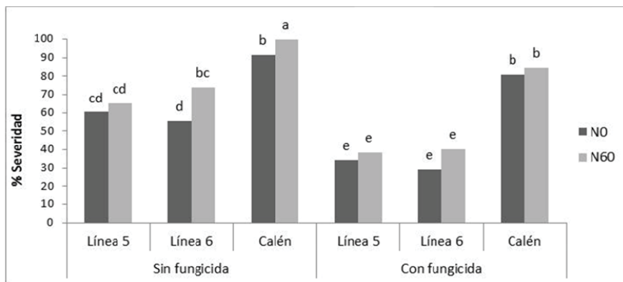
Figura 2: Medias de los valores de severidad (% Severidad) en EC8.2, para la interacción Fungicida x Fertilizante x Genotipos , de un ensayo con dos tratamientos de fungicidas, dos dosis de fertilización nitrogenada y tres genotipos de avena. Sin fertilizante (N0) y con 60 kgN.ha -1 (N60). Letras diferentes muestran diferencias significativas a través de los tratamientos (LSD, p < 0,05 ).
