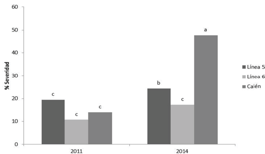
Figura 1: Medias de los valores de severidad (% Severidad) en EC3.9, para la interacción Año x Genotipos , de un ensayo con dos tratamientos de fungicidas, dos dosis de fertilización nitrogenada y tres genotipos de avena. Letras diferentes muestran diferencias significativas a través de los tratamientos (LSD, p < 0,05 ).
