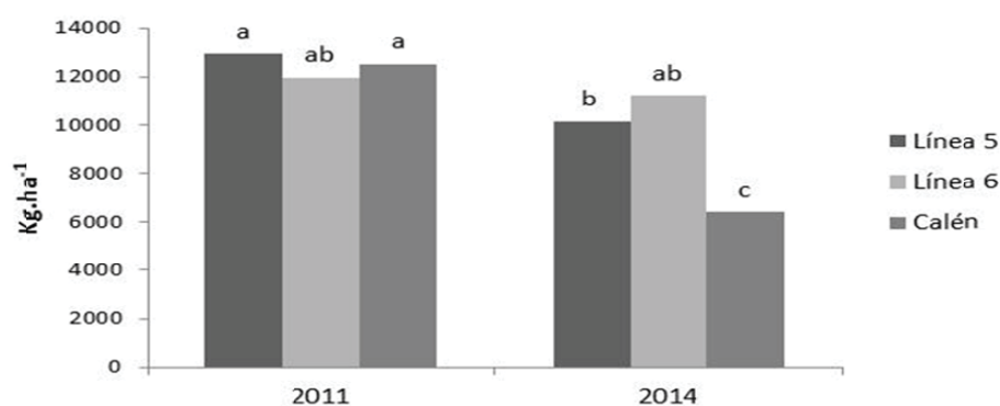
Figura 5: Media de los valores de biomasa aérea (Kg.ha -1 ) en EC8.2 para la interacción Año x Genotipos, en un ensayo con dos tratamientos de fungicidas, dos dosis de fertilización nitrogenada y tres genotipos de avena. Letras diferentes muestran diferencias significativas a través de los tratamientos (LSD, p < 0,05 ).
