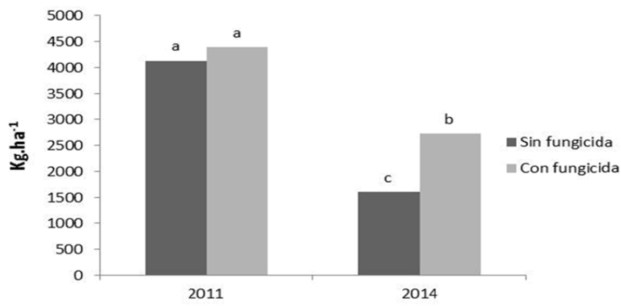
Figura 7: Media de los rendimientos (Kg.ha -1 ), para la interacción Año x Fungicida, de un ensayo con dos tratamientos de fungicidas, dos dosis de fertilización nitrogenada y tres genotipos de avena. Sin fungicida (SF) y con fungicida (CF). Letras diferentes muestran diferencias significativas a través de los tratamientos (LSD, p < 0,05 ).
