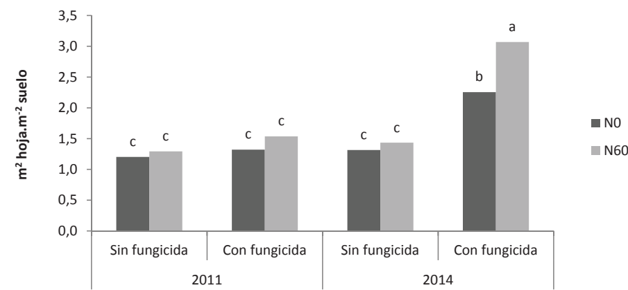
Figura 4: Media de los valores de IAF ( m^2 hoja. m^2 suelo) en EC8.2 para la interacción Año x Fungicida x Fertilizante, en un ensayo con dos tratamientos de fungicidas, dos dosis de fertilización nitrogenada y tres genotipos de avena. Sin fertilizante (N0) y con 60 \text{ kgN.ha}^{-1} (N60). Letras diferentes muestran diferencias significativas a través de los tratamientos (LSD, p < 0,05 ).
