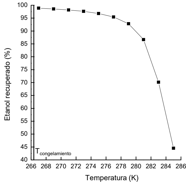
Figura 2.6 Recuperación de etanol en el permeado condensado vs temperatura de enfriamiento. Los datos de entrada corresponden a los presentados en la Tabla 2.4.
