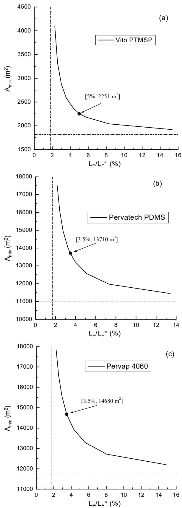
Figura 2.12 Mínima área de membrana ( \text{m}^2 ) en función de la relación del caudal de alimentación L_F/L_F^\infty (%) para las alternativas: (a) Vito PTMSP (experimentos a corto plazo), (b) Pervatech PDMS y (c) Pervap 4060. El punto señalado corresponde al valor de mínima área de membrana igual a 1.25 veces el valor asintótico horizontal.
