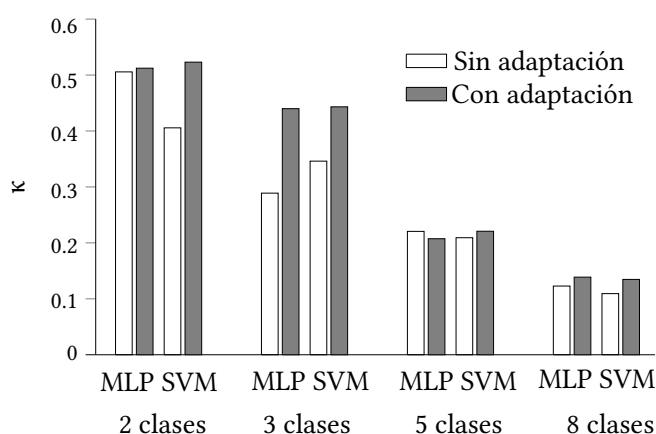
Figura 4.1: Resultados de la validación cruzada ( \kappa promedio) con el método de adaptación en reconocimiento de emociones categóricas. Se comparan registros de 2 a 25 minutos, conteniendo 2, 3, 5 y 8 emociones diferentes, con los clasificadores MLP y SVM.
